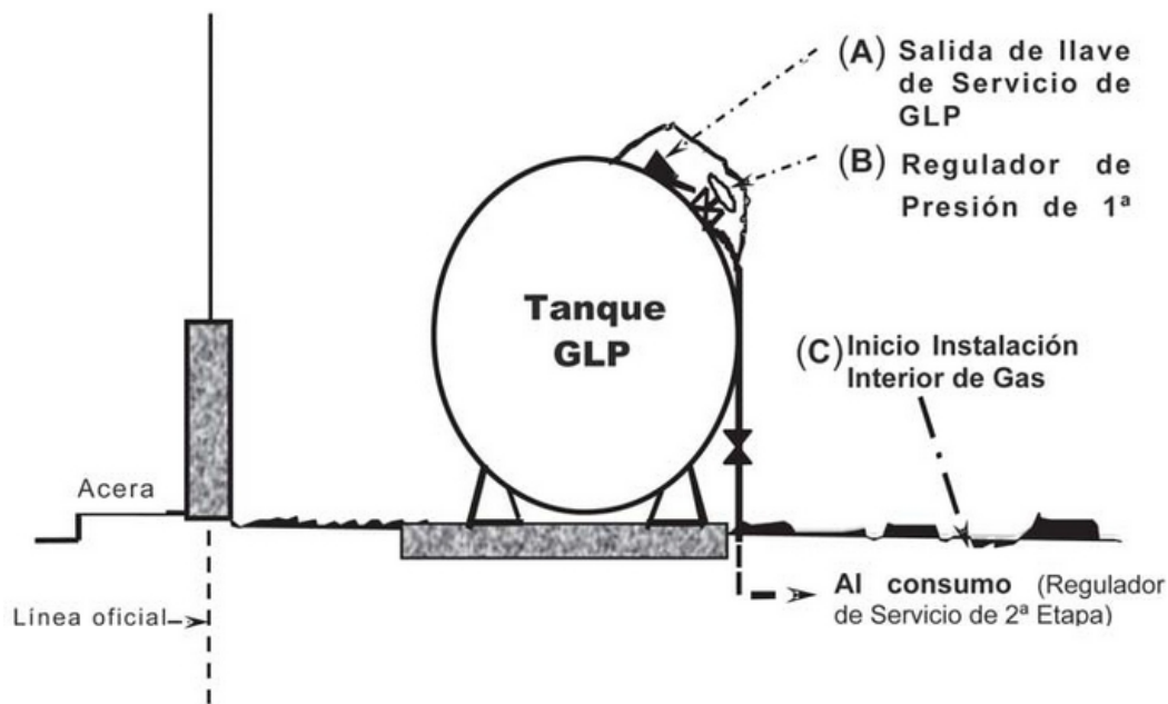
Figura 5. INSTALACIÓN INTERIOR DE GAS CON EQUIPO DE GLP.
