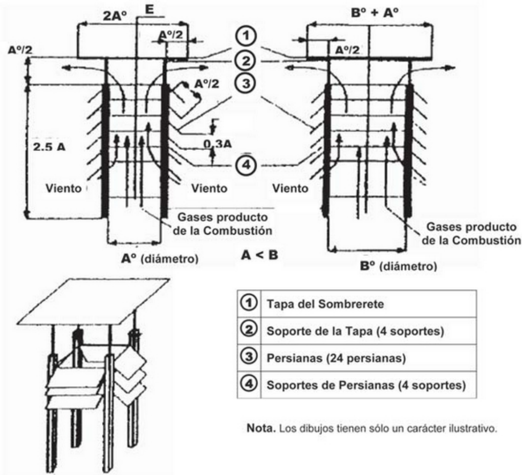
Figura 31. Sombbrero aspirador estacionario.
