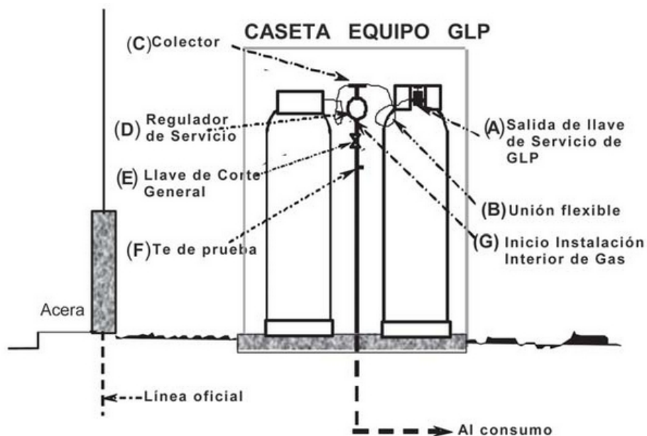
Figura 4. INSTALACIÓN INTERIOR DE GAS DE RED.
