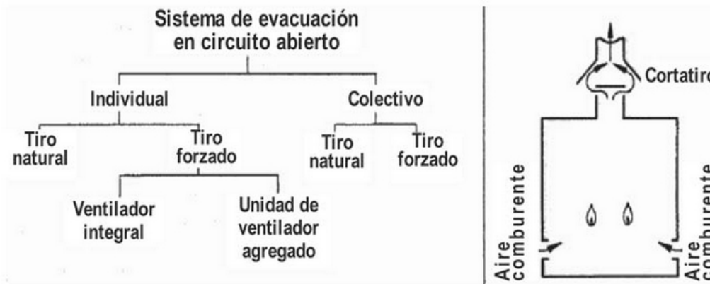
a.1 Sistema en circuito abierto, Figura 11.
