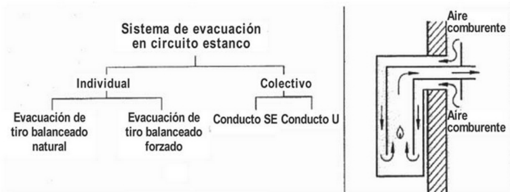
Sistemas de Evacuación - c) Circuito Estanco.
