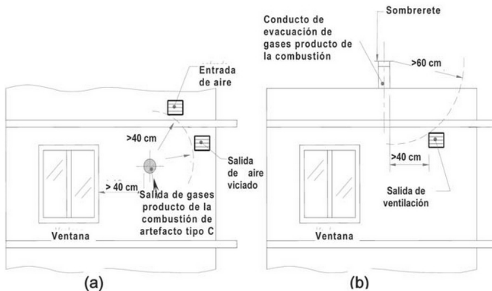
Figura 18. Distancias de las ventilaciones respecto de conductos de evacuación de gases.
