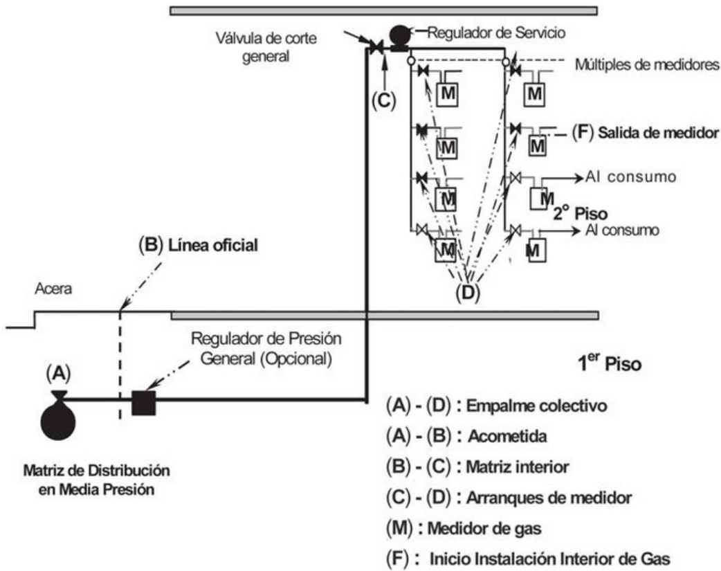
Figura 6. INSTALACIÓN INTERIOR DE GAS CON TANQUE DE GLP.
