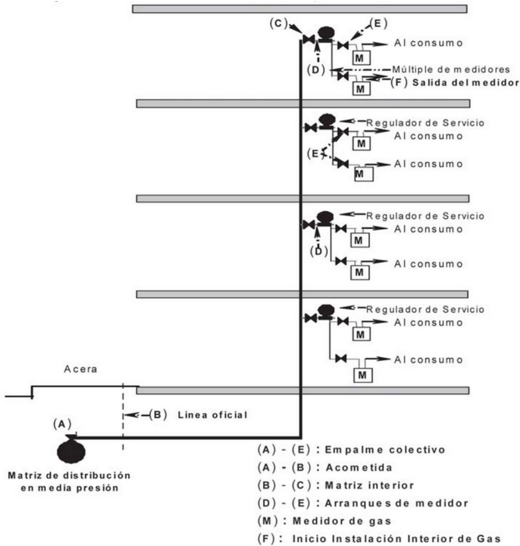
Figura 8. Instalación de Gas - Tipo Condominio.
