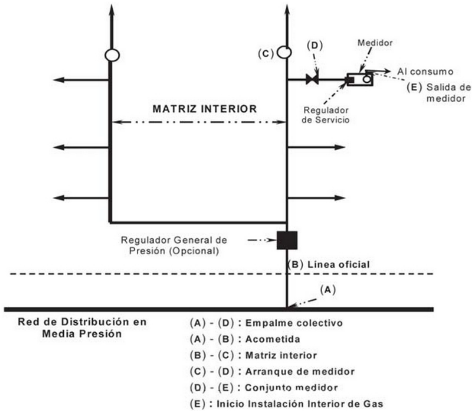
Figura 7. Instalación de Gas con Instalaciones Interiores.
